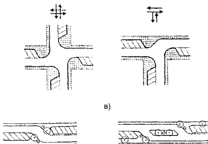
Рис. 11.10. Мероприятия по "успокоению движения" на участках дорог: а - изменение геометрии проезжей части (черным обозначена зона движения, белым - зона парковки), озеленение или другие элементы благоустройства; б - варианты изменения конфигурации пересечения и примыкания с размещением мест для парковки и зон пешеходного движения; в - варианты излома плана проезжей части с размещением мест для парковки
