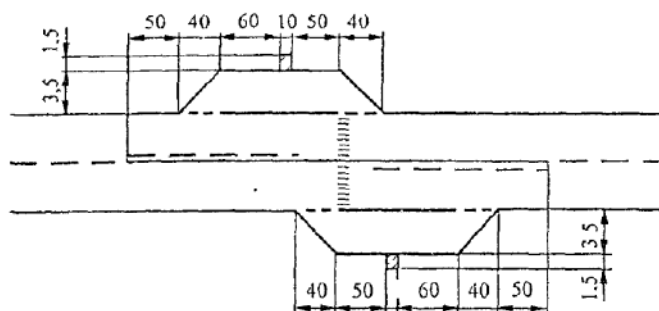
Рис. 11.9. Планировка автобусных остановок в населенных пунктах
