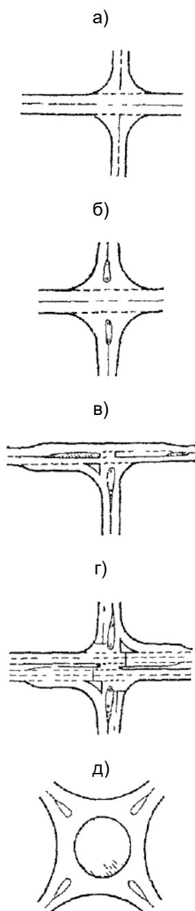
Рис. 8.2. Схемы планировочных решений пересечений: а - простое необорудованное пересечение; б - частично канализованное пересечение с направляющими островками
