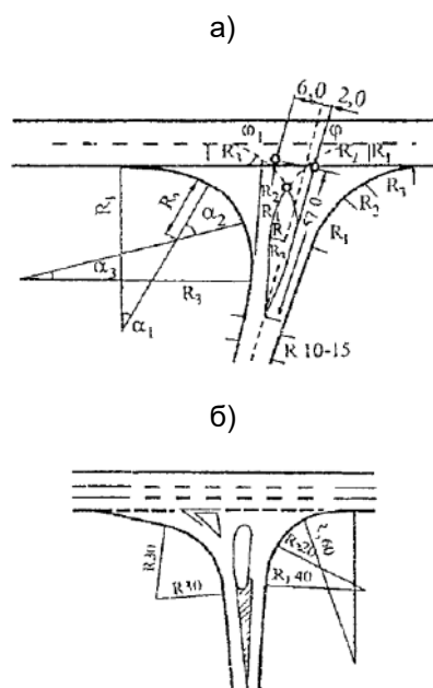
Рис. 8.10. Расположение островков на второстепенной дороге:
