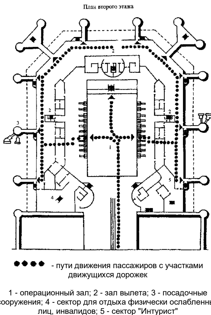
Рисунок В.13. Организация движения пассажиров в аэровокзале
